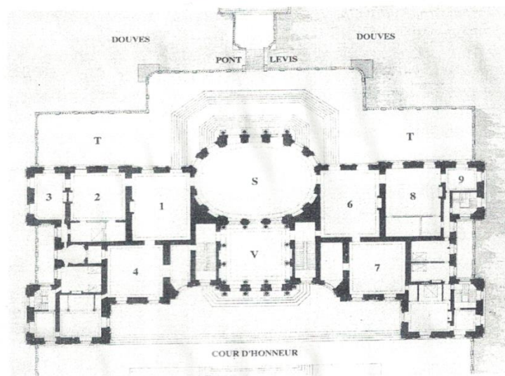
Plan de la distribution du rez-de-chaussée
